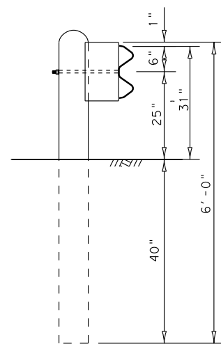
SECTION D-D
